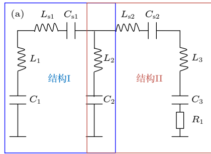
图 4 (a) 电磁诱导透明的等效电路模型; (b) 两种不同方法得到电磁诱导透明效应
