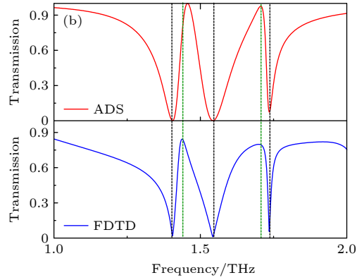
图 4 (a) 电磁诱导透明的等效电路模型; (b) 两种不同方法得到电磁诱导透明效应
