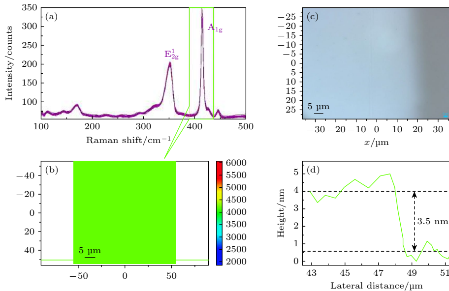
图 1 WS_2 纳米片的表征 (a) 532 nm 激光激发的拉曼光谱; (b) A_{1g} 模峰值强度的拉曼映射; (c) 光学显微光谱; (d) 原子力显微镜成像
