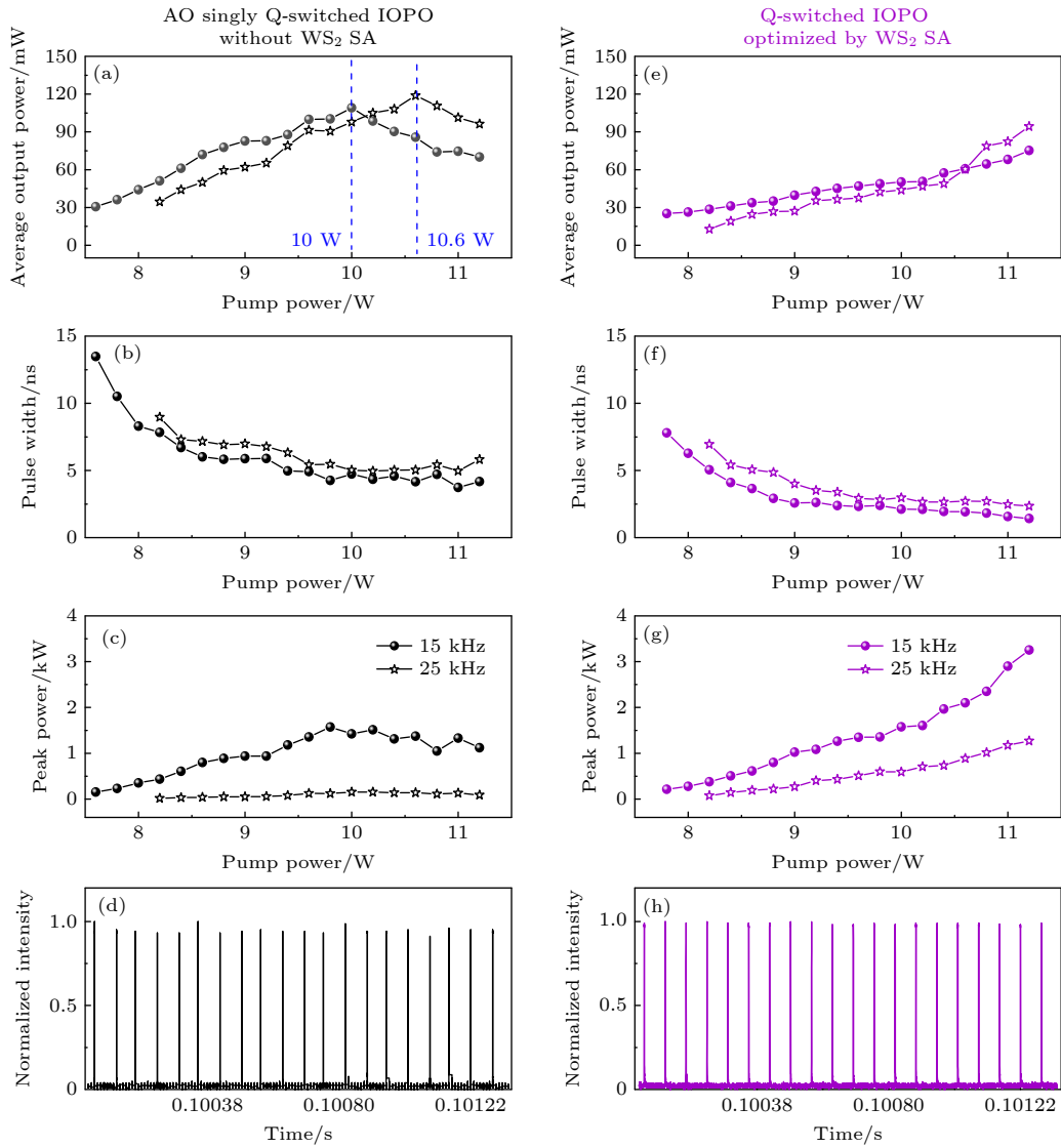
图 6 调 Q IOPO 的中红外闲频光输出特性 (a), (e) 平均输出功率; (b), (f) 输出脉冲宽度; (c), (g) 峰值功率; (d), (h) 输出脉冲序列. (a)–(d) AO 单调 Q IOPO 的输出结果; (e)–(h) WS_2 SA+AO 双调 Q IOPO 的输出结果 Fig. 6. Output characteristics of Q -switched IOPOs: (a), (e) Average output power; (b), (f) pulse width; (c), (g) peak power; (d), (h) pulse train; (a)–(d) output of AO Q -switched IOPO; (e)–(h) output of WS_2 SA+AO Q -switched IOPO.
