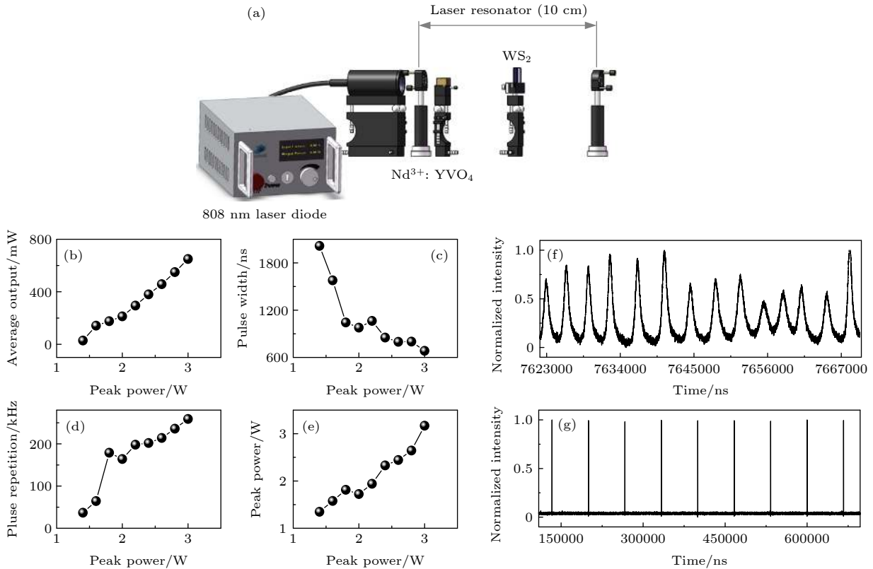
图3 WS 2 SA 被动调 Q 的 1.06 \mu\text{m} 激光 (a) 实验装置; (b) 平均输出功率; (c) 脉冲宽度; (d) 脉冲重复率; (e) 峰值功率; (f) WS 2 调 Q 、1.06 \mu\text{m} 脉冲波形; (g) WS 2 +AO 调 Q 的 1.06 \mu\text{m} 脉冲波形, f_p = 15 kHz
