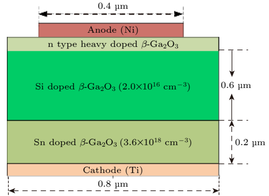
图 1 Ni/Ga 2 O 3 肖特基二极管的典型结构
