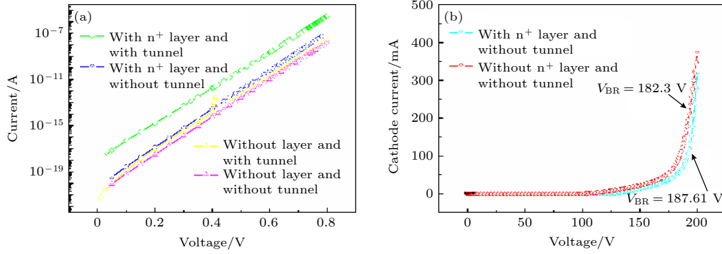
图 2 外延与未加 n^+ \beta - \text{Ga}_2\text{O}_3 薄层的肖特基性能曲线对比 (外延层厚度为 5 nm、浓度为 2.6 \times 10^{18} \text{ cm}^{-3} ) (a) 正向特性曲线; (b) 反向特性曲线
