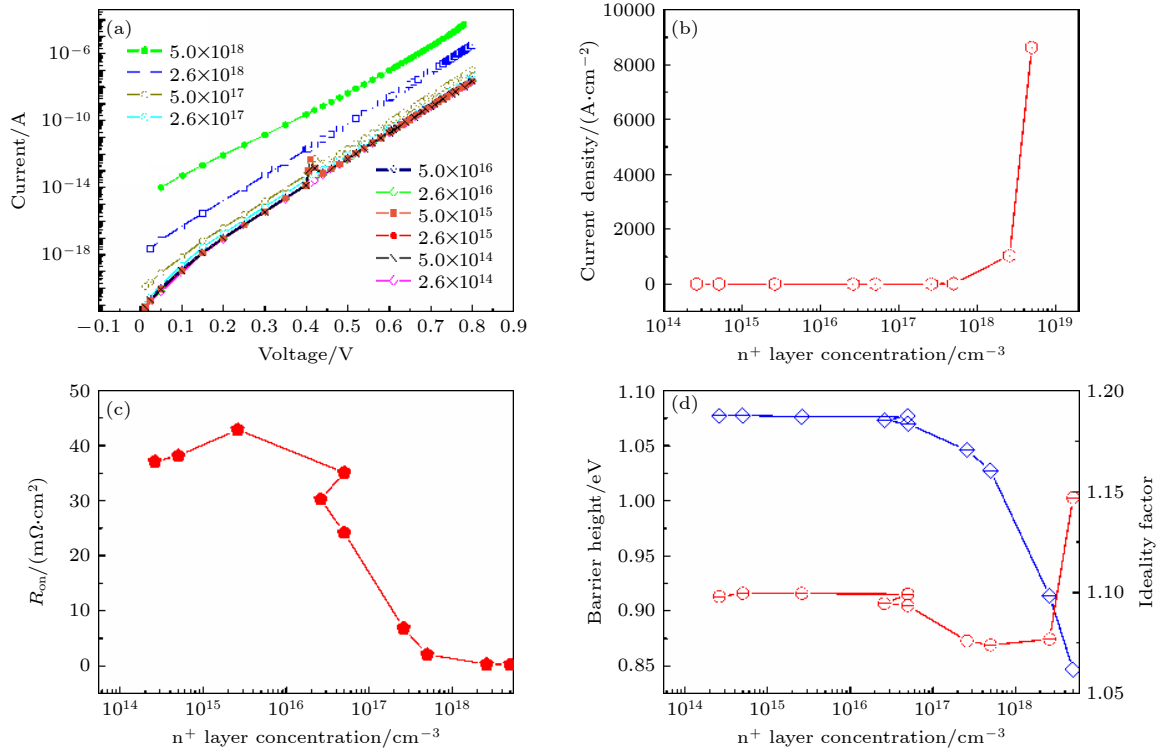
图 4 考虑隧穿效应, 在厚度为 5 nm 时, n^+ 层浓度对正向特性的影响 (a) 正向 I - V 曲线; (b) 0.8 V 正向偏置时, 电流密度与 n^+ 层浓度的关系; (c) 导通电阻与 n^+ 层浓度的关系; (d) 有效势垒高度和理想因子与 n^+ 层浓度的关系
