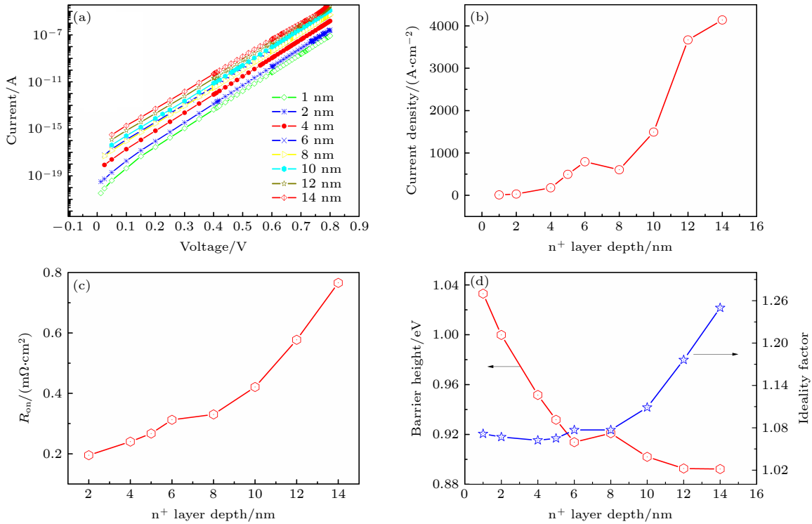
图3 考虑隧穿效应,在 2.6 \times 10^{18} \text{ cm}^{-3} 浓度下, n^+ 层厚度对正向特性的影响 (a)正向 I - V 曲线; (b) 0.8 V 正向偏置时,电流密度与 n^+ 层厚度的关系; (c) 导通电阻与 n^+ 层厚度的关系; (d) 有效势垒高度和理想因子与 n^+ 层厚度的关系
