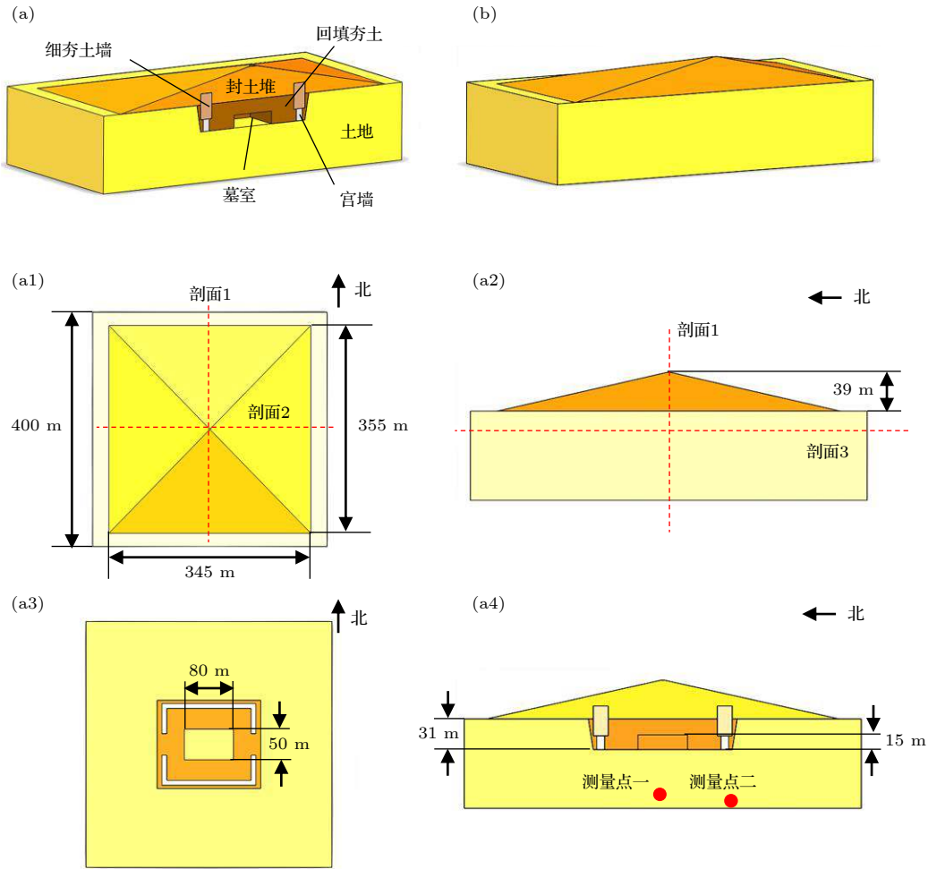
图 3 秦始皇陵模型示意图 (a) 模型 1 内部结构示意图; (a1) 模型 1 俯视图; (a2) 模型 1 正视图; (a3) 模型 1 剖面 3 示意图; (a4) 模型 1 剖面 1 示意图; (b) 模型 2 示意图 (无内部结构); Fig. 3. Model of Qinshihuang Mausoleum: (a) Inner structure of Model 1; (a1) top view of Model 1; (a2) front view of Model 1; (a3) profile 3 of Model 1; (a4) profile 1 of Model 1; (b) Model 2 (no inner structure).
