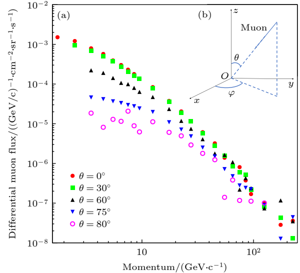
图1 (a) 实验测量得到的不同方向上的海平面 \mu 子通量 [20] ; (b) 探测器探测到的 \mu 子的方位角 \varphi 和天顶角 \theta , 其中 xOy 为水平面
