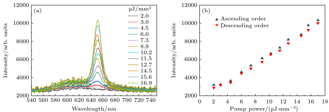
图 5 (a) Au/石墨烯激射样品在不同泵浦能量下的光致发光光谱; (b) 激射峰强度值与泵浦能量的关系图
