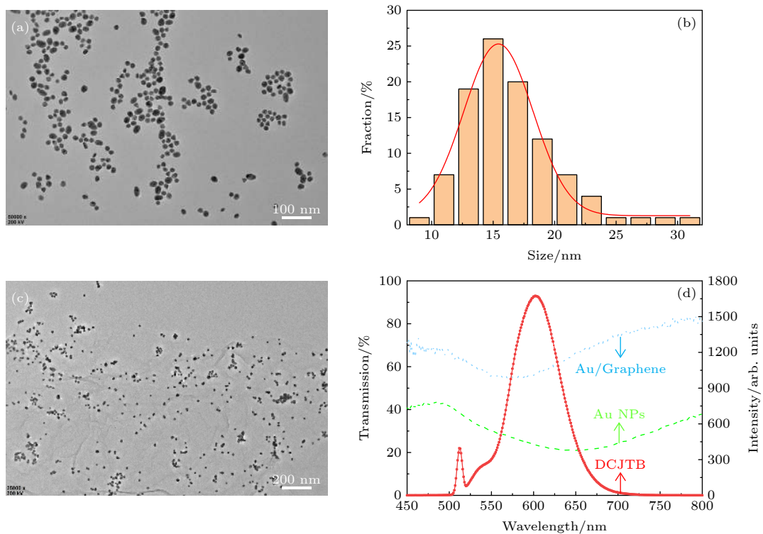
图 3 (a) Au 纳米颗粒的 TEM 图; (b) Au 纳米颗粒的粒径分布统计图; (c) Au/石墨烯的 TEM 图; (d) Au 纳米颗粒和 Au/石墨烯的透射光谱以及 DCJT 染料光致发光光谱
