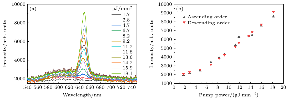
图 4 (a) Au 纳米颗粒激射样品在不同泵浦能量下的光致发光光谱; (b) 激射峰值与泵浦能量的关系图
