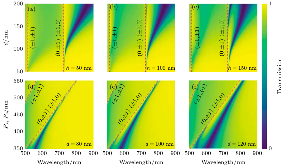
图 5 周期 P_x = P_y = 500 nm 保持不变, 对于银纳米圆柱高度 (a) h = 50 , (b) 100 与 (c) 150 nm 下直径 d 从 50 nm 变化到 200 nm 时阵列的透射谱. 高度 h = 100 nm 保持不变, 对于圆柱直径 (d) d = 80 , (e) 100 与 (f) 120 nm 下, 银纳米圆柱阵列周期 P 从 350 nm 变化到 550 nm 时的透射谱. 粉色虚线表示瑞利异常衍射阶次, 颜色条代表透射强度
