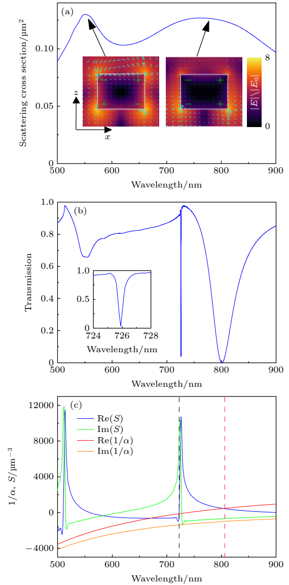
图 2 (a) 高度 h = 100 nm, 直径 d = 160 nm 的单个银纳米粒子散射截面光谱; 插图为偶极与四偶极 LSPRs 在 x - z 平面对应的电场强度与方向 (箭头) 分布, 纳米圆柱的侧面轮廓用白色框表示, “+”与“-”符号表示正负电荷; (b) 银纳米圆柱阵列在 x 偏振光照射下的透射谱, 插图为 QLPM 的放大图; (c) 银纳米圆柱阵列极化率倒数 ( 1/\alpha ) 与格点和 ( S ), 黑色虚线表示瑞利异常衍射, 粉色虚线表示 DLPM 共振波长
