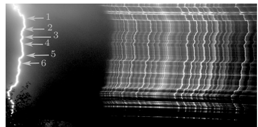
图1 闪电原始光谱图
