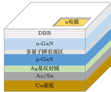
图 1 GaN 基 RCLED 器件结构示意图
