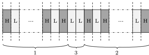
图 3 滤波器结构 DBR 的结构示意图 Fig. 3. Schematic illustration of Ta 2 O 5 /SiO 2 DBR with filter structure.
