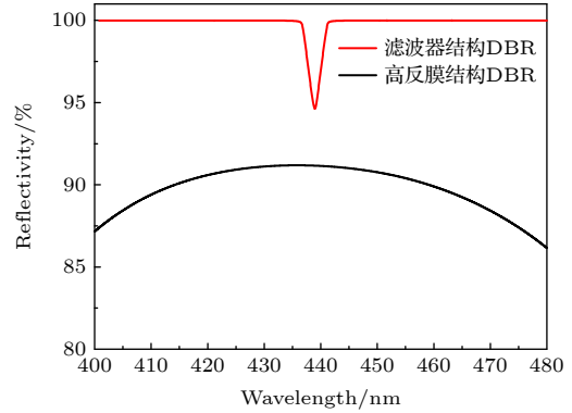
图9 高反膜结构DBR和滤波器结构DBR的反射率曲线测试结果
