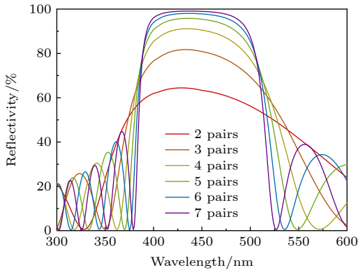
图 2 Ta 2 O 5 /SiO 2 高反膜结构 DBR 的反射率模拟曲线 Fig. 2. Simulated reflectivity spectra of Ta 2 O 5 /SiO 2 DBR with high-reflective-film structure.
