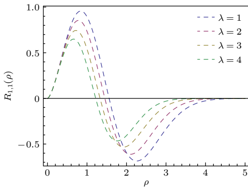
图 1 以 \rho 为变量取 4 个不同 \lambda 值的径向波函数
