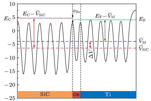
图 3 Ti/1GR/SiC 沿 z 轴的平均静电势
