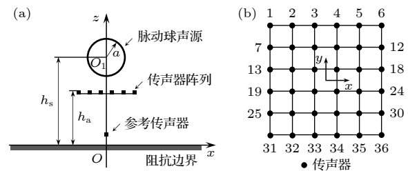
图 3 仿真声场示意图 (a) 脉动球声源、传声器阵列、参考传声器和阻抗边界的布置; (b) 阵列上传声器的编号
