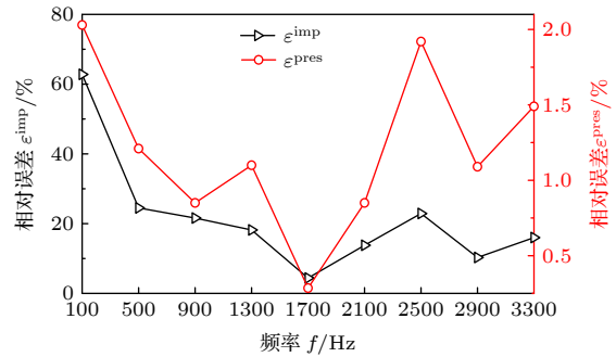
图 6 声阻抗率重构的相对误差 \epsilon^{\text{imp}} 和声源直接辐射声压重构的相对误差 \epsilon^{\text{pres}} 随频率 f 的变化曲线
