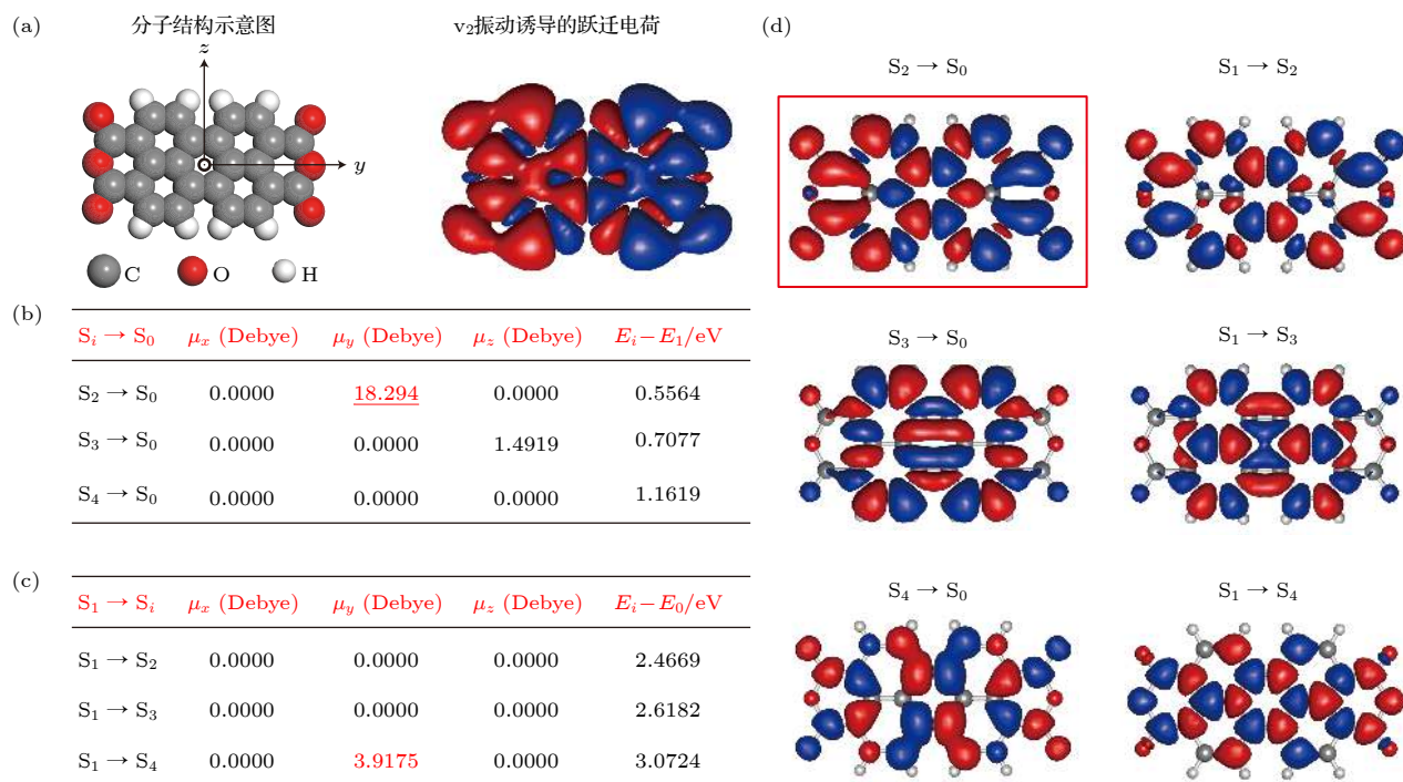
图 4 理论模拟的跃迁偶极矩和跃迁密度分布 (a) 左图为 PTCDA 分子结构示意图, 为方便与不同跃迁的跃迁密度进行比较, 右图再次展示了理论计算的 -2 价态的 PTCDA 分子的 v_2 模式振动诱导的跃迁电荷分布图; (b), (c) 理论计算的沿着 x , y 和 z 方向的不同电子态间的跃迁偶极大小以及对应能量差; (d) 理论模拟的不同电子态间跃迁的跃迁密度图
