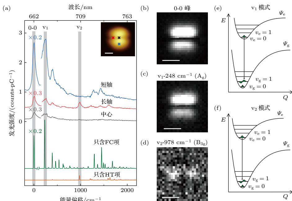
图2 位置依赖的STML光谱和特定振动峰的光谱成像 (a) 上面3条曲线分别为激发分子不同位置获得的STML光谱(+3 V, 20 pA, 60 s), 下面2条曲线分别为理论计算的FC项(绿色)和HT项(橘色)单独贡献的光谱; (b)–(d) 分别为0-0峰、 v_1 模式和 v_2 模式能量分辨的实空间光谱成像(+3.5 V, 30 pA, 每像素点3 s), 每条光谱均已扣除等离激元背景; (a)–(d) 比例尺均为1 nm; (e), (f) 基于DFT理论计算的 v_1 模式和 v_2 模式的势能曲线示意图
