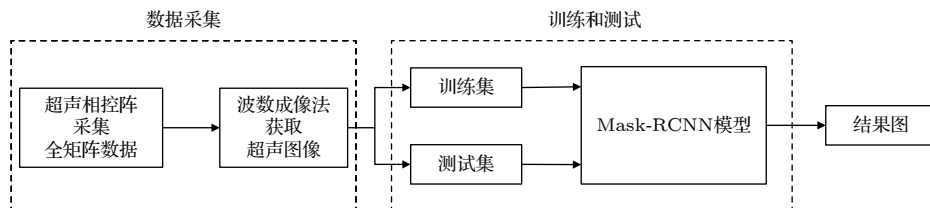
图 1 褶皱缺陷自动分类识别流程图
