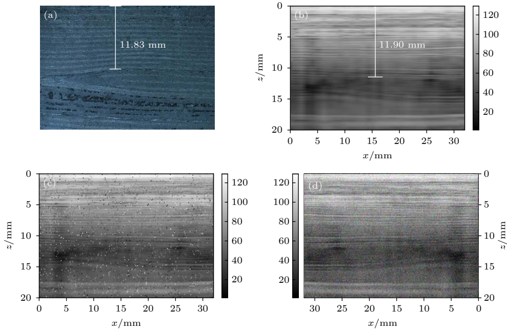
图 6 检测试样及其波数成像 (a) 显微镜图; (b) 波数成像法图; (c) 对图 (b) 加噪声; (d) 对图 (b) 调整亮度并沿 x 轴翻转 Fig. 6. est sample and its wavenumber imaging: (a) Microscope image; (b) wavenumber algorithm; (c) add noise to Figure (b); (d) adjust the brightness of Figure (b) and flip along the x -axis.
