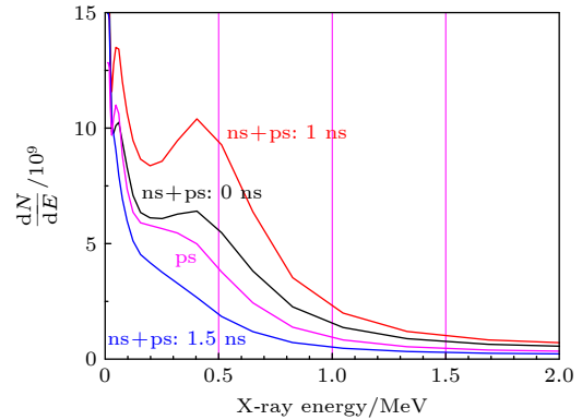
图 13 不同时间间隔条件下对应的伽马射线的能谱分布 Fig. 13. Spectrum distribution of gamma rays under different time interval.
