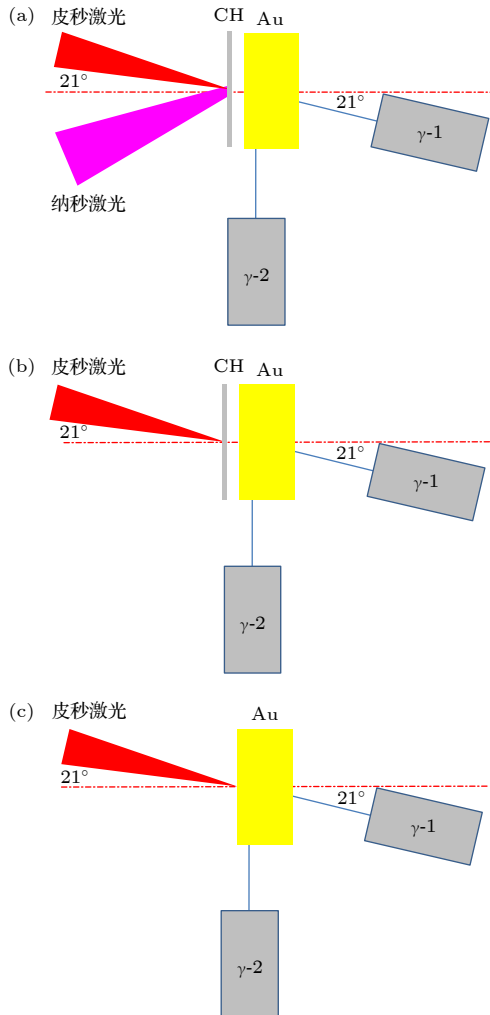
图 7 三种产生伽马射线的实验方案示意图 (a) 长短脉冲联合驱动双靶; (b) 单脉冲驱动双靶; (c) 单脉冲驱动单靶
