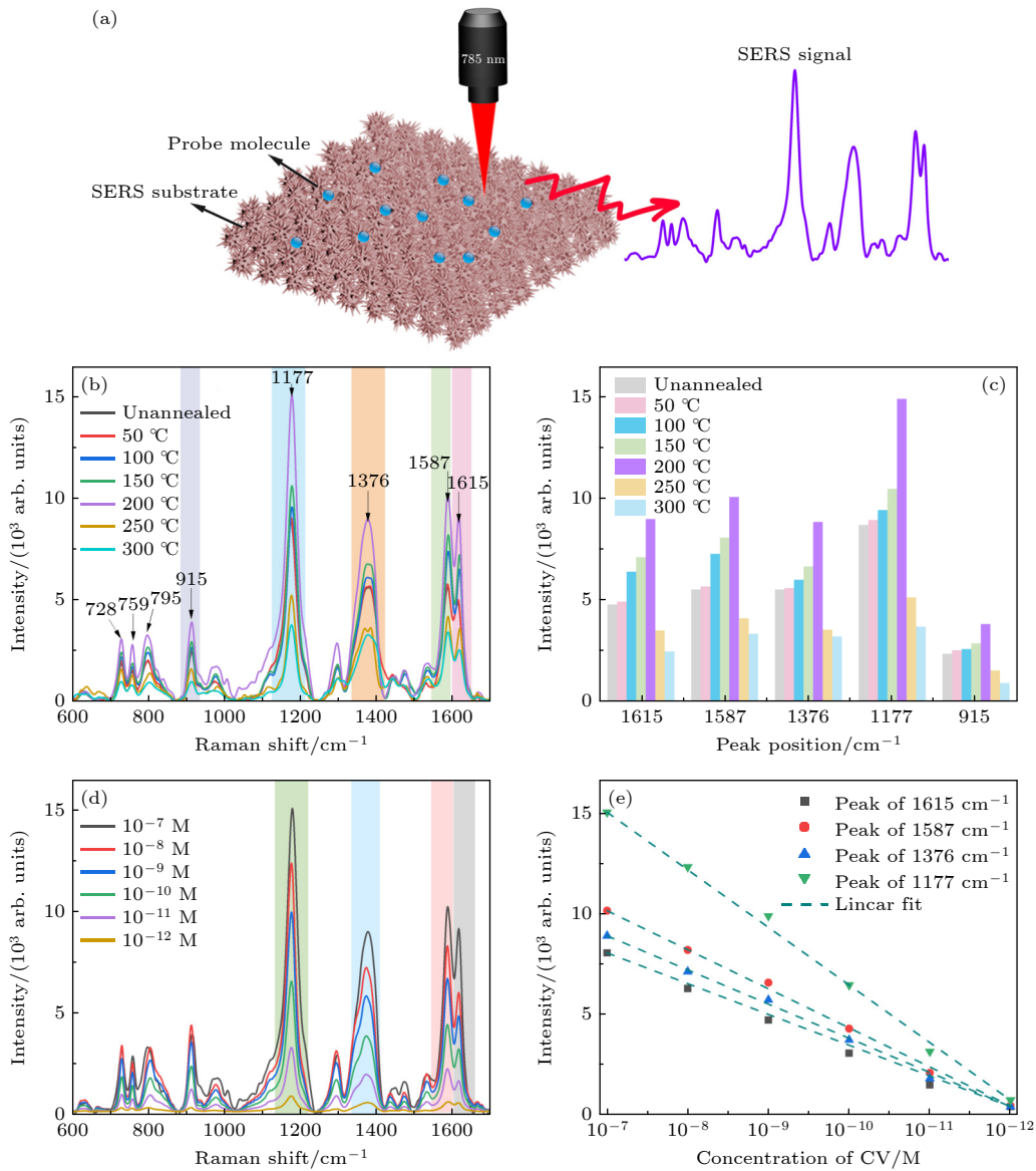
图 6 (a) SERS 信号采集示意图. 不同退火温度下, Au-Ag-Pt-Pd NUs 的 CV( 10^{-7} M) 拉曼信号谱图 (b) 和峰值的柱状图 (c). (d) 在退火 200 ^{\circ}\text{C} Au-Ag-Pt-Pd NUs 的 SERS 基底上, 不同浓度 CV 分子的 SERS 谱图. (e) 探针分子 CV 位于 1177, 1376, 1587 和 1615 \text{cm}^{-1} 特征峰的 SERS 信号强度与 CV 分子浓度的线性关系
