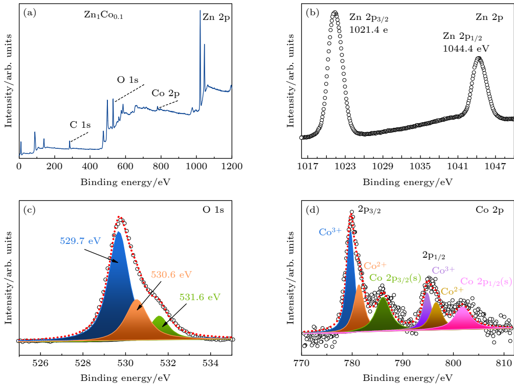
图 4 Zn 1 Co 0.1 复合微结构的 XPS 图谱 (a), Zn 2p (b), O 1s (c) 和 Co 2p (d) Fig. 4. XPS spectra of Zn 1 Co 0.1 composite microstructure (a), Zn 2p (b), O 1s (c) and Co 2p (d).
