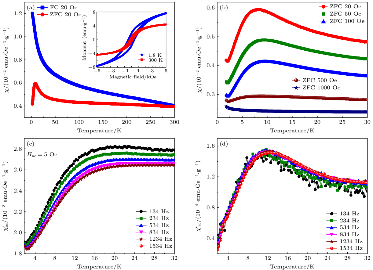
图 4 掺杂样品 K_3DPF-A 的 PPMS 磁性测试结果 (a) K_3DPF-A 在外磁场 20 Oe 下的 ZFC 和 FC 直流磁化率测试曲线, 插图为 M-H 曲线; (b) K_3DPF-A 在不同磁场下的 ZFC 曲线; (c) K_3DPF-A 交流磁化率曲线的实部; (d) K_3DPF-A 交流磁化率曲线的虚部
