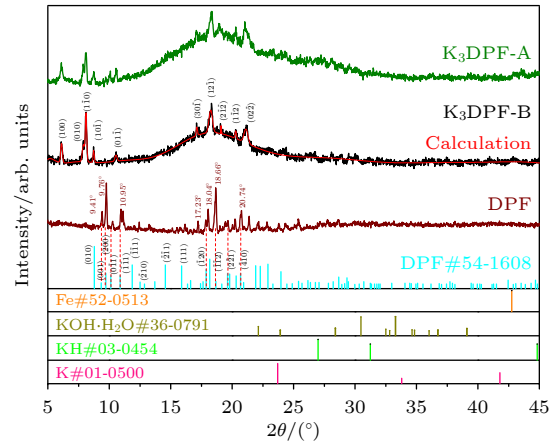
图 8 纯 DPF 和 275 °C 退火下钾掺杂 DPF 的 XRD 图谱 Fig. 8. The XRD patterns of pristine and potassium-doped tris(diphenacyl)iron annealed at 275 °C.
