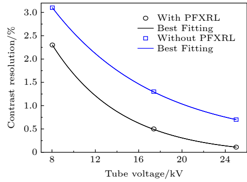
图 7 对于测量的水模, 在使用和不使用 PFXRL 下的 Micro-CBCT 系统对比度分辨率与管电压的关系 Fig. 7. Measured contrast resolution of Micro-CBCT system as a function of tube voltages for water phantom.
