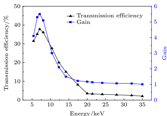
图5 PFXRL的传输效率和能量密度增益随X射线能量的依赖关系
