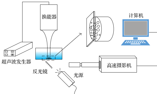
图 5 实验装置示意图
