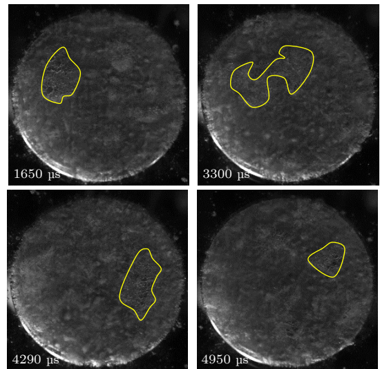
图 6 薄层液体中的空化结构
