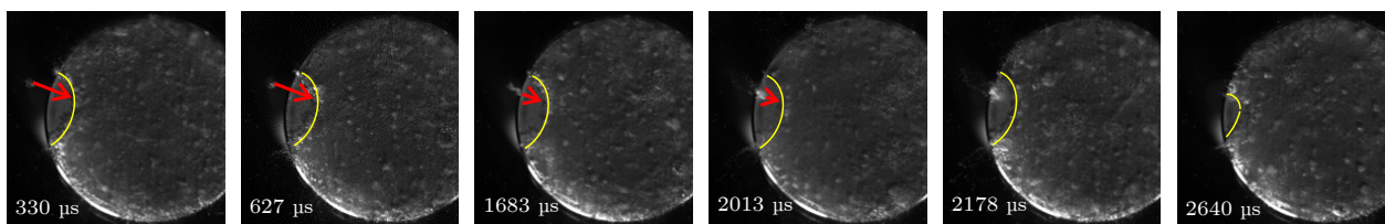
图 8 气泡云吸引周围气泡团
