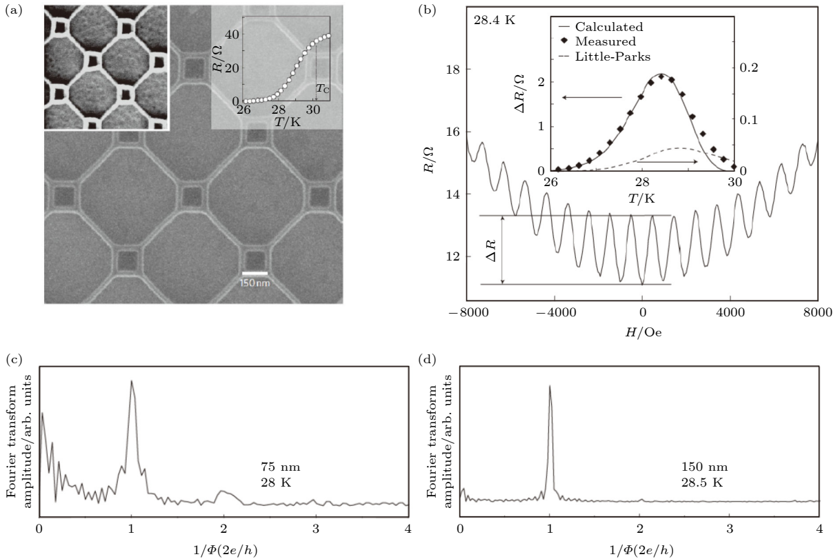
图 7 热激发的磁通涡旋运动导致的磁电阻振荡效应 [87] (a) 高温超导 \text{La}_{1.84}\text{Sr}_{0.16}\text{CuO}_4 纳米结构的扫描电子显微镜照片, 该结构由两个互相嵌套、成角 45^\circ 的正方形构成, 右上角的插图为电阻-温度关系以及据此定义的临界温度 T_C ; (b) 磁电阻的振荡现象, 其中磁电阻的振荡幅度用 \Delta R 表示. 内置插图为振荡幅度 \Delta R 与温度的关系 (散点图), 该振幅远远大于利特尔-帕克斯效应的预测 (断续线), 却与根据热激发的磁通涡旋的运动模型计算的结果 (实线) 相吻合; (c), (d) 对振荡曲线作傅里叶变换得到的幅度-磁通倒数关系. 其中 (c), (d) 分别对应于 75 nm, 150 nm 边长的小正方形. 变换后只能在 2e/h 位置处看到一个尖锐的峰, 而理论预测的 e/h 和 4e/h 峰并不显著 (图中 4e/h 位置的矮峰源于 2e/h 的二倍频信号, 并不是本征性质的反映)
