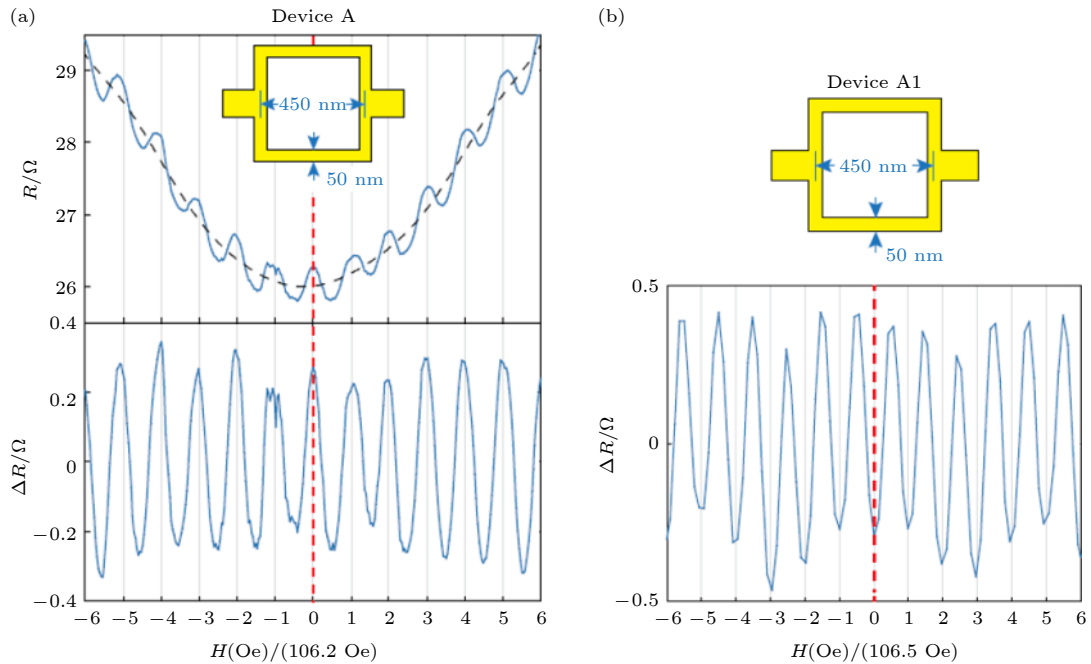
图4 对 \alpha -BiPd超导环的利特尔-帕克斯振荡的分析 [75] (a) 零磁通对应于磁电阻极大的利特尔-帕克斯振荡原始曲线(上图,标记为 R )及去掉多项式背景后的结果(下图,标记为 \Delta R ),该振荡的行为与图3(b)相对应,这样的超导环被称为“ \pi ”环; (b) 零磁通对应于磁电阻极小的利特尔-帕克斯振荡,这里直接展示的是去掉背景后的结果(标记为 \Delta R ),与图3(a)相对应,这样的超导环被称为“0”环
