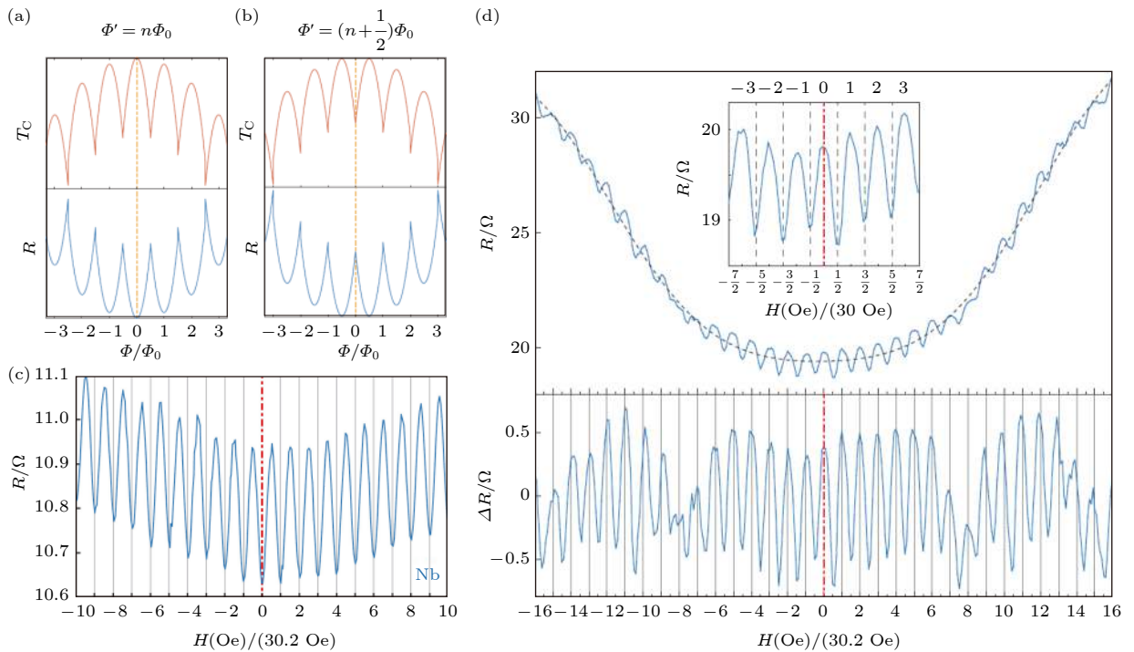
图 3 常规超导体 (s 波配对) 与自旋三重态超导体配对机制对应的利特尔-帕克斯效应对比 [66] (a) 常规超导体的温度 (上图)、磁电阻 (下图) 随磁场变化的利特尔-帕克斯振荡示意图, 零磁通状态对应于临界温度 T_C 的极大值、磁电阻 R 的极小值; (b) 自旋三重态配对的超导体的温度 (上图)、磁电阻 (下图) 随磁场变化的利特尔-帕克斯振荡示意图, 零磁通状态对应于 T_C 的极小值和 R 的极大值, 与 (a) 刚好相反; (c) 常规超导体 Nb 磁电阻的利特尔-帕克斯振荡效应, 与图 (a) 相符, 其中磁场强度对 30.2 Oe (单个磁通线对应的磁场强度, 1 \text{ Oe} = 10^3/(4\pi) \text{ A/m} ) 进行了归一化处理; (d) 拓扑超导体 \beta\text{-Bi}_2\text{Pd} 磁电阻的利特尔-帕克斯振荡, 上图为原始曲线, 下图为去掉多项式背景信号后的曲线, 其振荡现象与图 (b) 相符, 证实了其自旋三重态配对的物理机制
