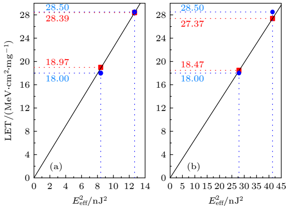
图 9 不同波长下器件发生 SEB 的 E_{\text{eff}}^2 与 LET 关系对比图 (a) 620 nm; (b) 720 nm
