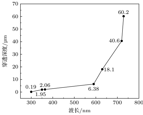
图3 不同波长下激光在 GaN 材料中的穿透深度 Fig. 3. Laser penetration depth in GaN materials at different wavelengths.
