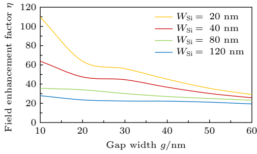
图 3 仿真计算的不同波导间隙的硅基混合表面等离子光场窄化器件的场增强因子
