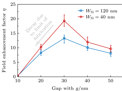
图6 实验加工的不同波导间隙的硅基混合表面等离子激元光场窄化器件的场增强因子
