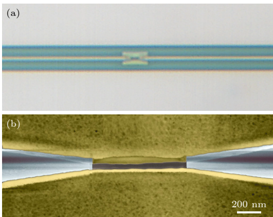
图 4 实验加工的硅基混合表面等离子光场窄化器件 ( W_{Si} = 120 nm, g = 30 nm, h_m = 30 nm) 的 (a) 光学显微镜图和 (b) SEM 图 (伪彩上色)
