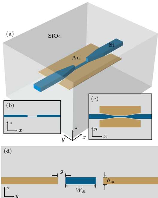
图 1 硅基混合表面等离子激元光场窄化器件的结构示意图 (a) 三维图; (b) 侧视图; (c) 俯视图; (d) 中间处的截面图 Fig. 1. Schematic of the proposed silicon hybrid plasmonic nanofocusing device: (a) 3D perspective view; (b) side view; (c) top view; (d) cross-sectional view at the center.
