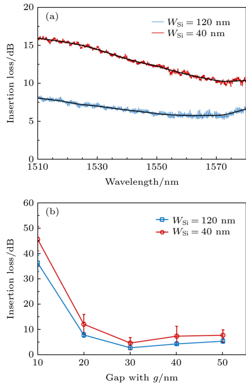
图 5 (a) 实验加工的硅基混合表面等离子光场窄化器件的损耗谱线; (b) 不同间隙宽度 g 对应的损耗
