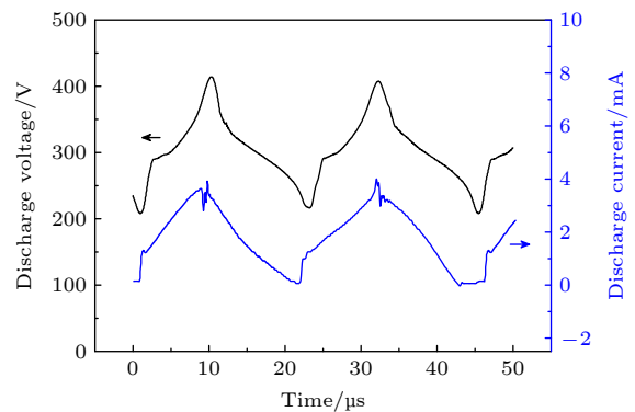
图 4 放电电压和电流波形
