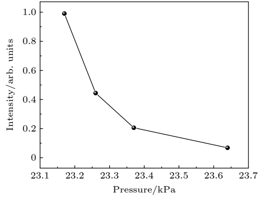
图 10 加入氮气对主要发射线 696.543 nm 的影响 (a) 23.17 kPa; (b) 23.26 kPa; (c) 23.37 kPa; (d) 23.64 kPa
