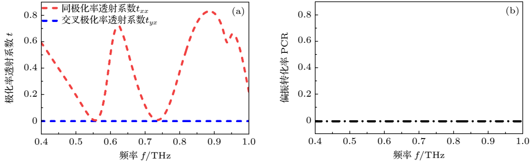
图 4 偏振仿真结果 (a) 透射系数; (b) 偏振转化率
