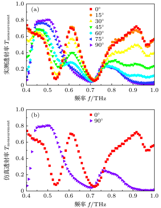
图 7 THz-TDS 系统测量结果 (a) 0°—90°; (b) 0°与 90°
