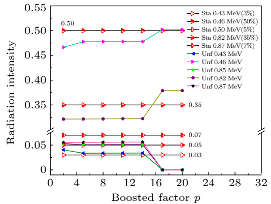
图 9 不同 p 值下标准相对强度数据与反演数据的对比 Fig. 9. The comparison of the standard relative intensity data and the unfolded data at different p -values.
