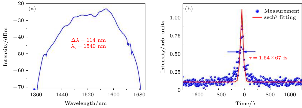
图 4 拉锥光纤 WS 2 SA 被动锁模掺铒光纤激光器的实验结果 (a) 脉冲光谱, 中心波长 1540 nm 的 3 dB 带宽为 114 nm; (b) 脉冲宽度为 67 fs [48]
