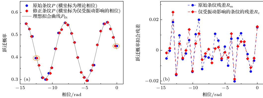
图 12 第 1 组实测数据 (a) 修正前后的干涉条纹与理论拟合曲线 (典型修正点用橘色圆圈标出), (b) 原始残差与计算出的仅由振动导致的条纹残差
