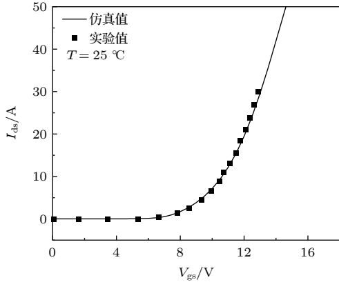
图 7 实验与仿真转移特性曲线对比
