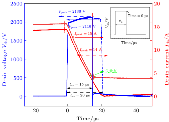
图 2 单脉冲 UIS 测试失效前最后一次实验波形 (划线) ( L_{load} = 3.3 mH, t_{av} = 20 \mu s, E_{av} = 0.33 J) 与单脉冲 UIS 测试失效实验波形 (实线) ( L_{load} = 3.3 mH, t_{av} = 15 \mu s, E_{av} = 0.37 J)
