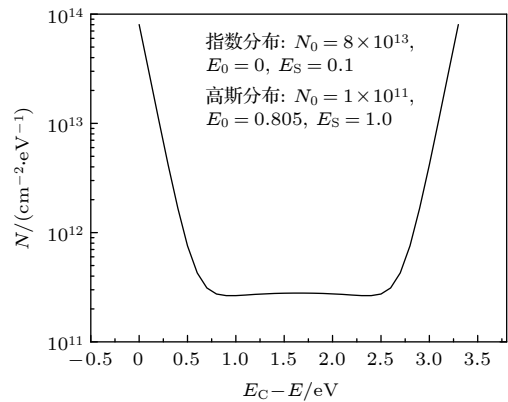
图 6 界面态密度在禁带中的分布 Fig. 6. SiC/ SiO_2 interface state density profile used in this simulation.
