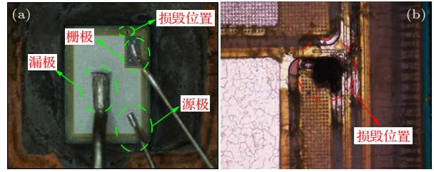
图 3 UIS 测试失效后拆封的双沟槽 4H-SiC MOSFET (1200 V/80 m \Omega ) 俯视图 (a) 4H-SiC 功率 MOS 器件压焊点; (b) UIS 测试 DUT 失效时 SEM 图
