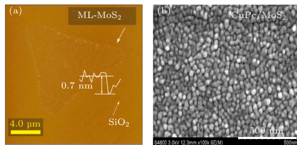
图 2 CuPc/MoS 2 异质结的形貌表征 (a) 单层 MoS 2 的 AFM 图; (b) CuPc/MoS 2 异质结的 SEM 图
