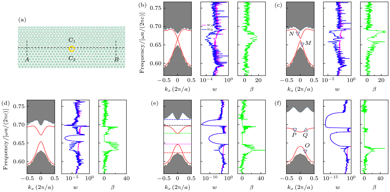
图 4 (a) 模型结构示意图; (b)—(f) 当 D=0.13a 时, 分别取 r 值为 0.01a, 0.02a, 0.04a, 0.06a 和 0.08a 时系统的投影边界态以及赝自旋光波在边界处的单向传输效果图, 左侧图: 投影边界态, 中间图: 光波能量 w_A 和 w_B , 右侧图: 单向隔离率 \beta ; (e) 中蓝、黑、绿、洋红、红色虚线 (由上至下) 分别对应上体态带底、上边界态带顶、上边界态带底、下边界态带顶和下体态带顶处的频率位置; (c) 中 M 和 N 两点分别对应频率 0.648 的下边界态和频率 0.684 的上边界态; (f) 中 O 点对应频率 0.622 的下边界态、 P 和 Q 点对应频率 0.685 的两上边界态
