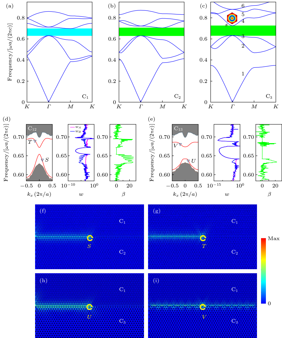
图 9 (a)—(c) C_1, C_2 和 C_3 结构光子晶体的频带结构, (c) 中插图为其第 4 个频带 \Gamma 点处的本征模场 |E_z| ; (d) 和 (e) C_{12} 结构和 C_{13} 结构的赝自旋螺旋边界态及其单向传输效果图. 左侧图: 投影边界态, 中间图: 光波能量 w_A 和 w_B , 右侧图: 单向隔离率 \beta . (f)—(i) 分别对应 C_{12} 结构中赝自旋光源激发的 (d) 图中 S 点和 T 点边界态以及 C_{13} 结构中赝自旋光源激发的 (e) 图中 U 点和 V 点边界态在界面处的传播
