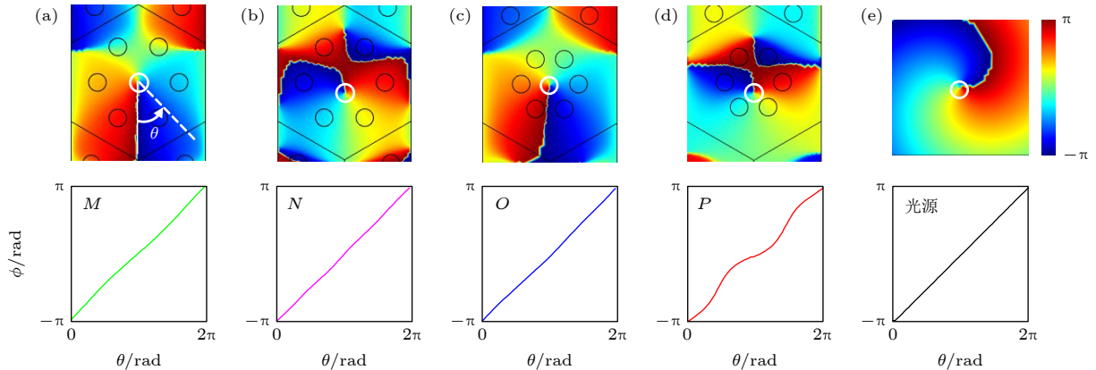
图 8 上行图边界处激发光源附近本征场 E_z 的相位分布 (a)–(d) 分别对应图 4(c) 中 M , N 点和图 4(f) 中 O , P 点边界态相位分布; (e) 自由空间中赝自旋光源的电场相位分布. 下行各图对应上行各图中白色圆圈路径上的光场的相位变化, 激发光源位于白色圆圈中心
