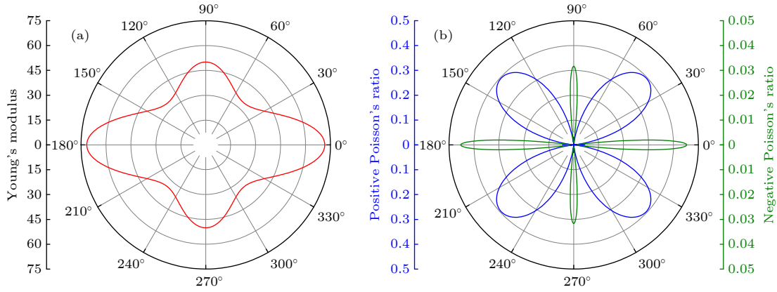
图 2 SiGeS 的 (a) 杨氏模量及 (b) 泊松比
