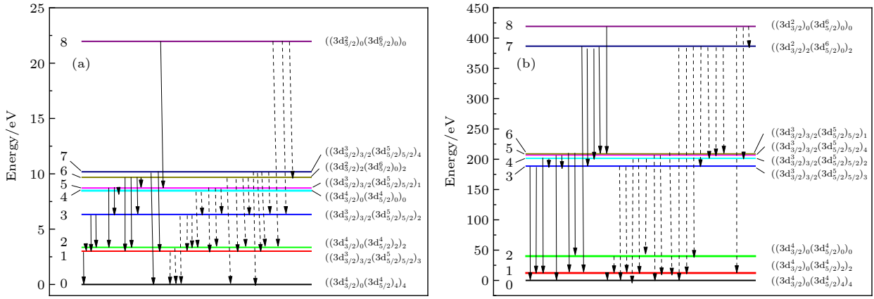
图 2 类铁钼 ( \text{Mo}^{16+} ) 离子 (a) 和铀 ( \text{U}^{66+} ) 离子 (b) 基组态内的禁戒跃迁, 其中实线为 M1 跃迁, 虚线为 E2 跃迁, 图中的数字 (0, 1, 2, ...) 表示能级序号
