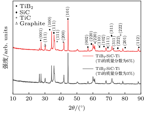
图 4 TiB 2 -SiC-Ti(Ti 的质量分数为 3%) 和 TiB 2 -SiC-Ti (Ti 的质量分数为 6%) 烧结样品的 X 射线衍射图谱
