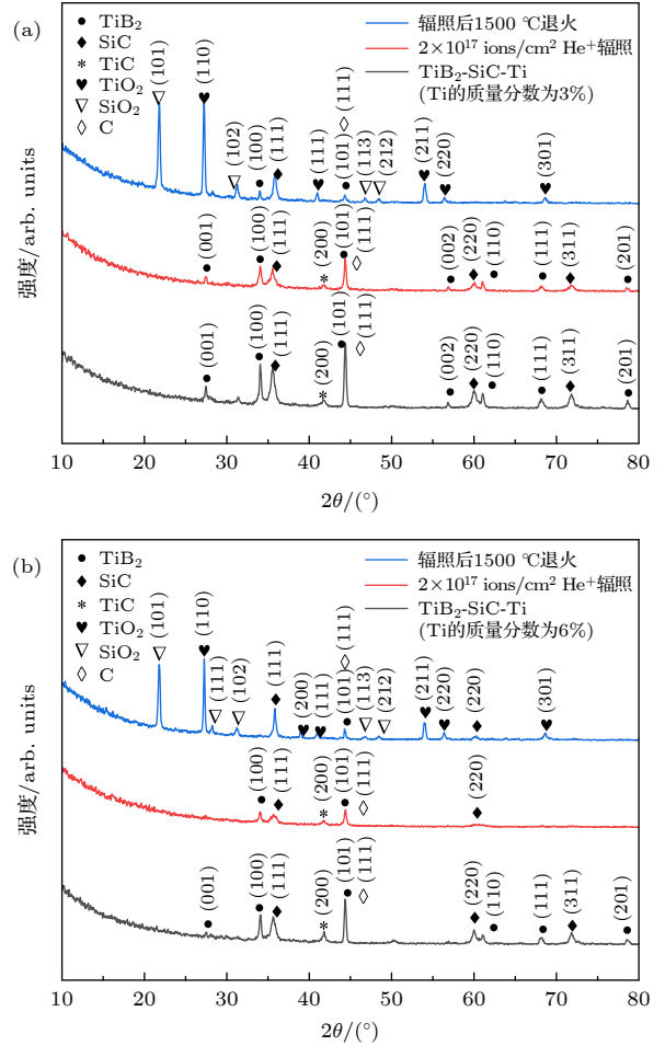
图 5 0.5°入射角下 TiB 2 -SiC-Ti(Ti 的质量分数为 3%) (a) 和 TiB 2 -SiC-Ti(Ti 的质量分数为 6%) (b) 样品的 X 射线衍射图谱, 包括原始状态、室温下 60 keV, 2 \times 10^{17} ions/cm 2 He + 辐照以及辐照后 1500 °C 退火 3 种条件
