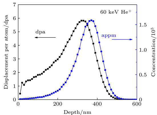
图 1 SRIM 模拟 60 keV, 2 \times 10^{17} ions/cm 2 \text{He}^+ 辐照 \text{TiB}_2\text{-SiC-Ti} 复合材料得到的损伤深度分布及 He 原子浓度深度分布图
