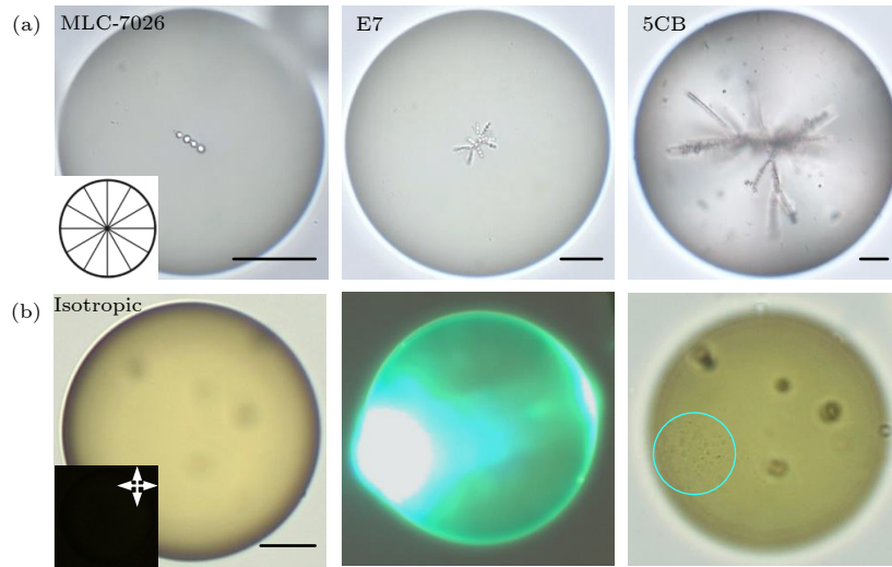
图 4 液晶种类和相态对激光注射的影响 (a) 液晶材料弹性系数 K 值越高, 注入难度越大; (b) 激光辅助机械注射针对各向同性的材料依然有效 (标尺 20\ \mu\text{m} )
