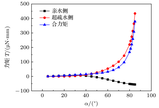
图 8 力矩 T 与 \alpha 的关系
