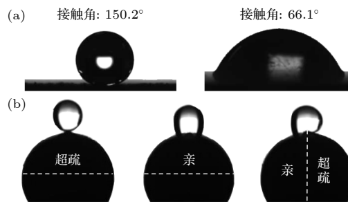
图 1 (a) 与 Janus 颗粒相同处理步骤下的超疏水平板和亲水平板的接触角; (b) 液滴滴在 Janus 颗粒不同润湿性表面的状态
