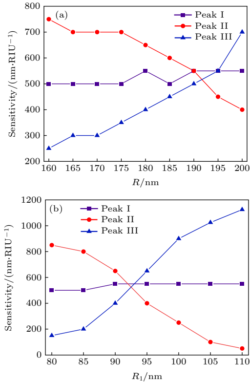
图 7 3 个峰的灵敏度随参数 R 和 R_1 的变化 Fig. 7. Sensitivity trends of the three peaks with different parameters R and R_1 .
