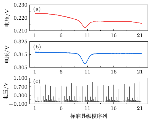
图 2 吸收信号对比 (a) 光束 4 引入前获得的水分子吸收信号; (b) 光束 4 引入后获得的水分子吸收信号; (c) F-P 标准具纵模信号
