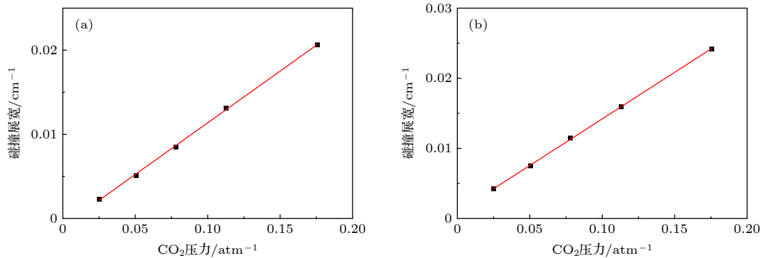
图 4 Voigt 线型 (a) 和 qSDV 线型 (b) 拟合后, 不同气压下的碰撞展宽值 (1 atm = 1.01 × 10 5 Pa)
