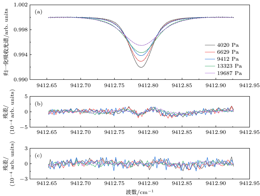
图 3 (a) 9412.790 cm -1 处, 不同压力下的测量点及拟合结果; (b) 使用 voigt 线型拟合吸收光谱得到的残差; (c) 使用 qSDV 线型拟合吸收光谱得到的残差
