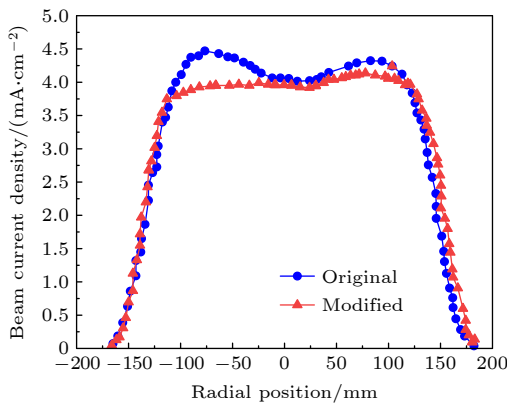
图 14 栅极热稳定设计优化前后束流密度分布
