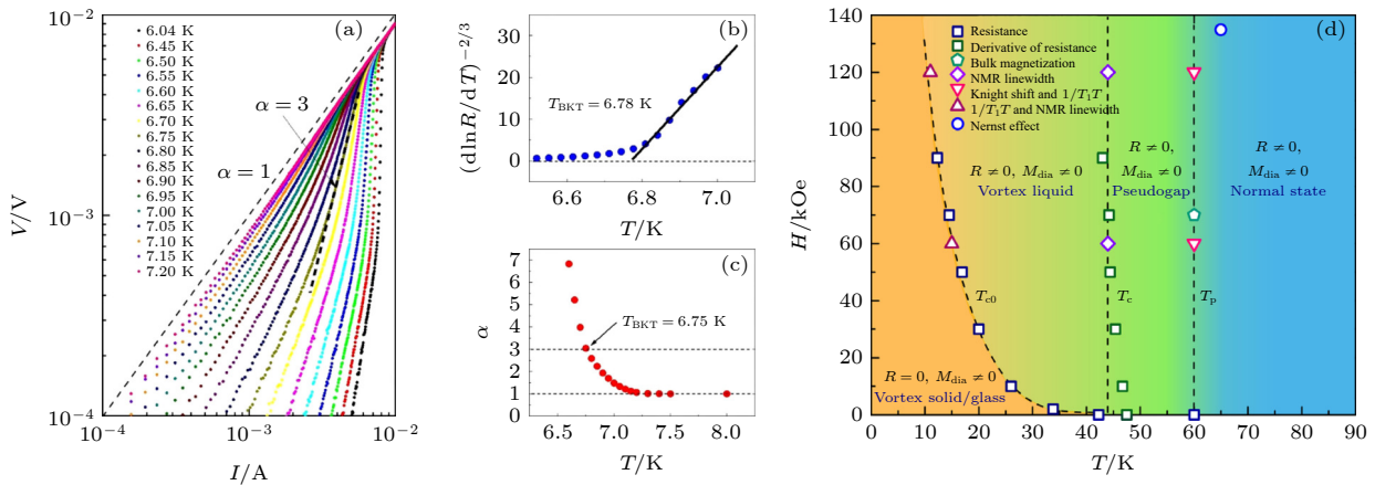
图 4 (CTA) x SnSe 2 中的二维超导与 (TBA) x FeSe 中的赝能隙相图 (a) (CTA) x SnSe 2 在超导转变温度附近的 I-V 曲线 [26] ; (b) (CTA) x SnSe 2 的 R(T) 曲线, 其中纵坐标是 (d \ln R / dT)^{-2/3} [26] ; (c) 从 (CTA) x SnSe 2 的 I-V 曲线中分离出来的幂指数 \alpha ; (d) (TBA) x FeSe 的磁场-温度相图, 其中 T_{c0} 是零电阻温度, T_c 是通过 NMR 谱线展宽和电阻曲线一阶微分定义的超导转变温度, T_p 是电子预配对的温度 [13]
