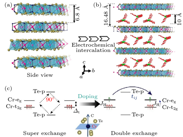
图 2 \text{Cr}_2\text{Ge}_2\text{Te}_6 中插层 \text{TBA}^+ 分子后的结构和磁作用机制变化 (a), (b) \text{Cr}_2\text{Ge}_2\text{Te}_6 插层 \text{TBA}^+ 分子前后的结构示意图 [25] ; (c) \text{Cr}_2\text{Ge}_2\text{Te}_6 插层 \text{TBA}^+ 分子前 (左图) 和插层 \text{TBA}^+ 分子后 (右图) 的磁性作用机制示意图 [25]
