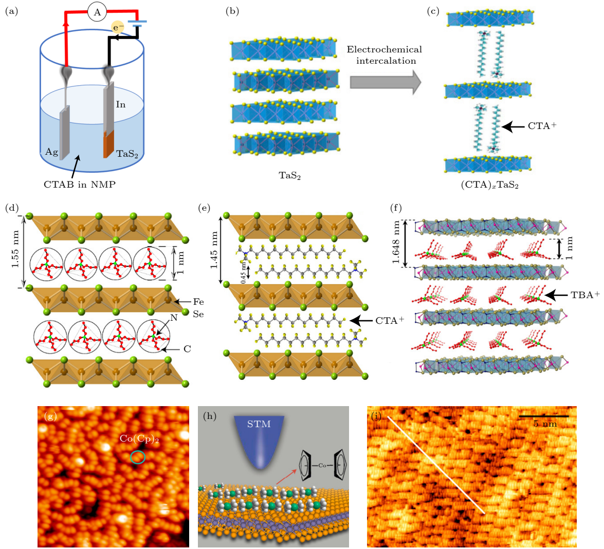
图 1 电化学有机分子插层的过程及结构演化 (a) 电化学电解池的结构及电荷流动示意图, 包括工作电极 (固定有二维材料的 In 丝)、对电极 (Ag 片) 和电解液 (溶有季铵盐的有机溶液); (b), (c) CTA + 插层 TaS 2 前后的结构示意图, 其中有有机分子 CTA + 垂直于 TaS 2 的 ab 面 [11] ; (d), (e), (f) (TBA) x FeSe [12] , (CTA) x FeSe [13] 以及 (TBA) x Cr 2 Ge 2 Te 6 [25] 的结构示意图, 其中 TBA + 在层间单层排列, CTA + 在层间以双层平行排列; (g), (h) (Cp) 2 Co 插层 SnSe 2 的 STM 形貌图和其对应的结构示意图, 有机分子 (Cp) 2 Co 的五元环平面与 SnSe 2 的 ab 面垂直 [18] ; (i) (CTA) x FeSe 的 STM 形貌图, 其中 CTA + 分子在 FeSe 层间紧密排列, 且 CTA + 分子的长链与 FeSe 的 ab 面平行 [13]
