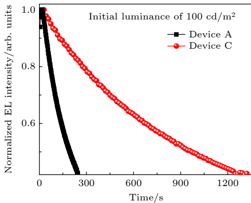
图 5 器件 A 和器件 C 的工作稳定性 Fig. 5. Working stability of device A and device C.
