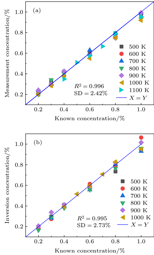
图 5 各温度下光谱探测的 C_2H_2 浓度与配气时所记录的浓度对比 (a)(b) 分别为有无颗粒物的测量环境
