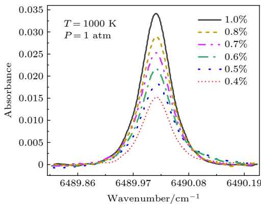
图 4 1000 K 温度下测得的不同浓度的 C_2H_2 直接吸收光谱信号
