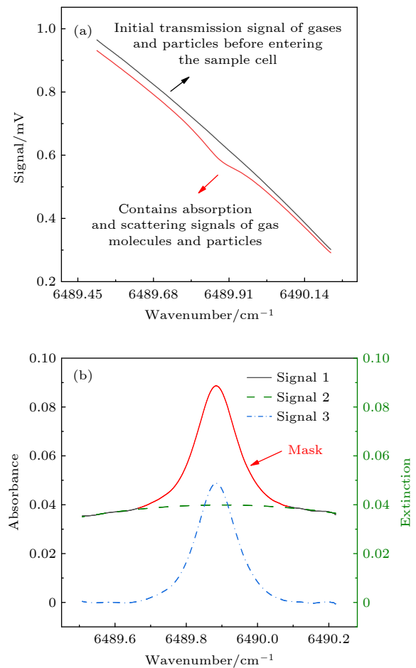
图 3 (a) 气体吸收和颗粒物消光信号; (b) 信号处理
