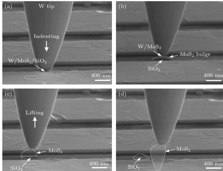
图 3 MoS 2 /SiO 2 vdWHs 纳米压痕过程典型的 SEM 图 (a) W 探针压入形成 W/MoS 2 /SiO 2 vdWHs; (b) MoS 2 纳米片被 W 探针黏附从 SiO 2 /Si 基底剥离形成鼓包; (c) MoS 2 纳米片发生不完全穿透断裂; (d) MoS 2 纳米片解理撕裂后, 最终与 SiO 2 /Si 完全分离
