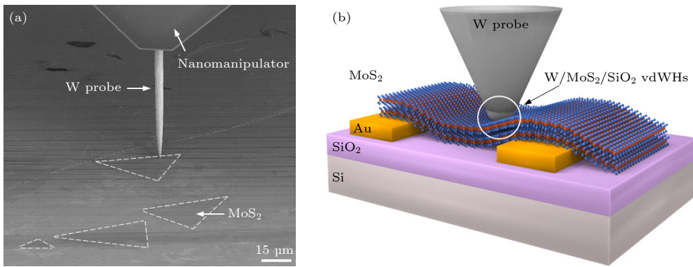
图 2 (a) W 探针和 MoS 2 纳米片 SEM 图像; (b) MoS 2 /SiO 2 vdWHs 纳米压痕实验示意图
