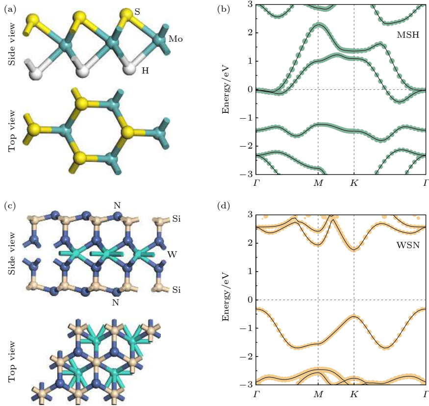
图 1 (a) MSH 与 (c) WSN 的侧视图与俯视图; (b) MSH 与 (d) WSN 的能带结构. 费米能级被设置为 0 点 Fig. 1. Top and side views of (a) MSH and (c) WSN; band structures of (b) MSH and (d) WSN. The Fermi level is set to zero.
