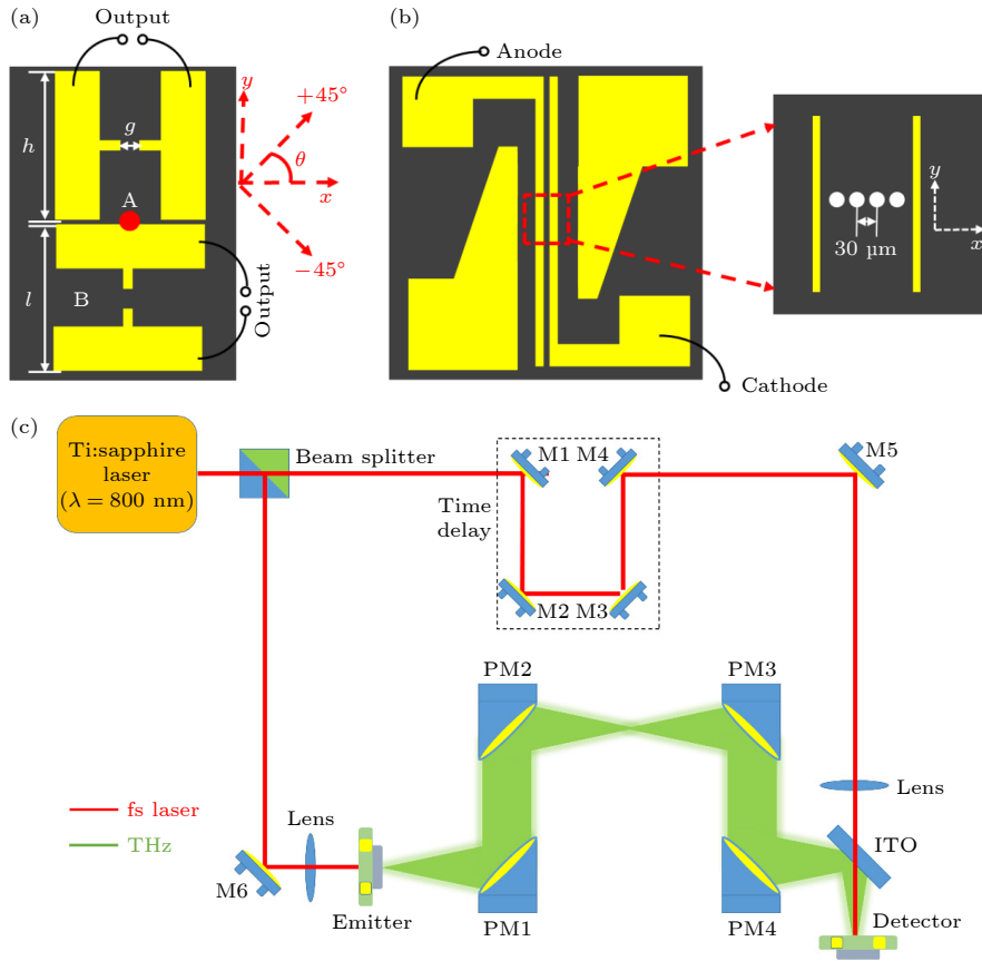
图 1 (a) PTHD 结构; (b) THz 波辐射天线结构; (c) THz-TDS 光路示意图
