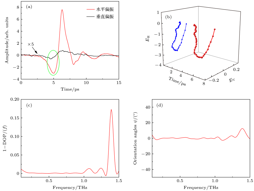
图 3 (a) 水平和垂直偏振的 THz 时域信号; (b) 图 (a) 绿色圆圈部分的 THz 脉冲的空间轨迹; 与频率相关的 (c) DOP 和 (d) THz 电场方位角
