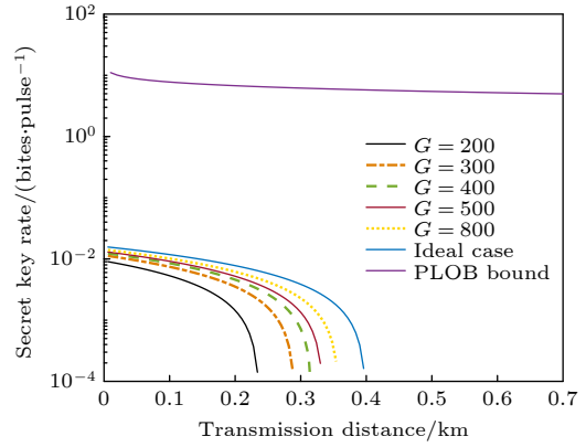
图 4 在对称情况以及不同的 PSA 增益参数 G 下所提出方案的安全密钥率与传输距离的关系
