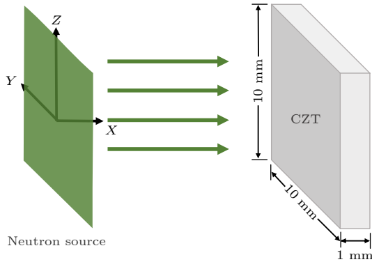
图 2 Geant4 几何模型结构示意图
