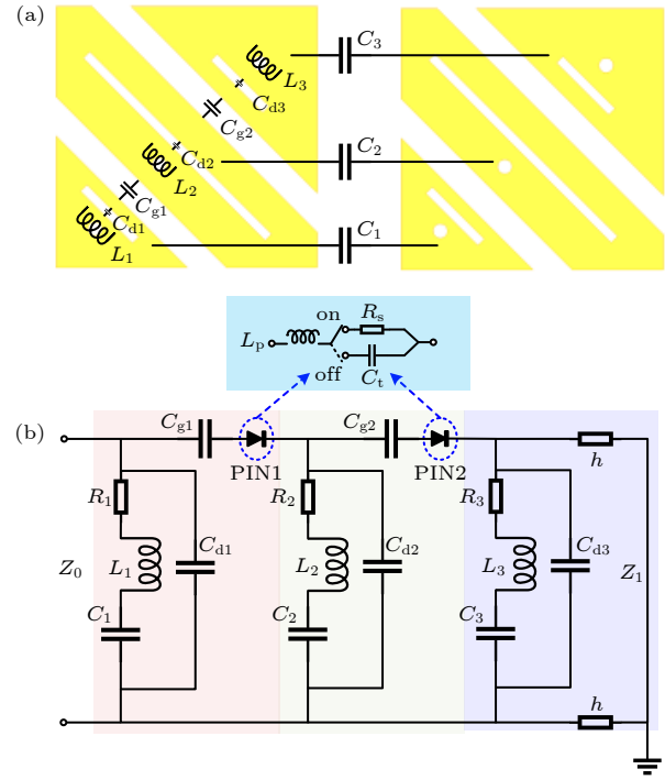
图 2 等效电路 (a) 等效电路分析; (b) 等效电路模型
