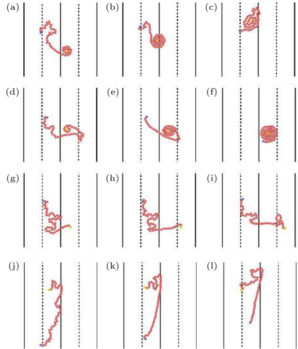
图 4 柔性链跨区域运动的快照 ( d = 8 ) (a)—(c) 第一种跨区域运动模式, 即头部从非活性区进入活性区, 很快形成螺旋并最终返回非活性区; (d)—(f) 第二种跨区域运动模式, 即头部从非活性区进入活性区, 在大部分链段进入活性区后形成螺旋并最终在活性区形成完整螺旋; (g)—(i) 第三种跨区域运动模式, 即头部从非活性区进入活性区, 并跨越整个活性区进入下一个非活性区; (j)—(l) 第四种跨区域运动模式, 即中间部分从非活性区进入活性区造成其后面的链段产生明显的 (沿纵向即 y 方向的) 拉伸
