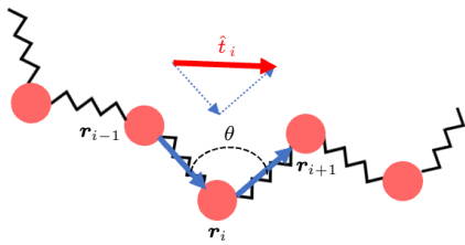
图 2 活性力示意图
