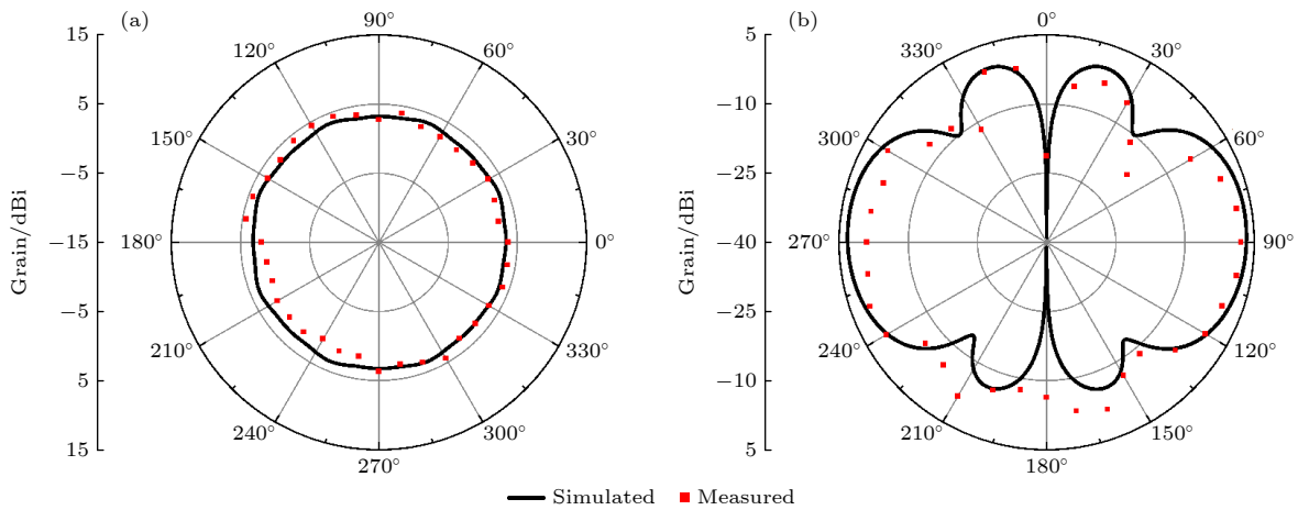
图 11 全向波束增益方向图 (a) xoy 面; (b) yozy 面
