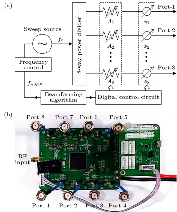
图 7 射频馈电网络 (a) 原理图; (b) 实物图
