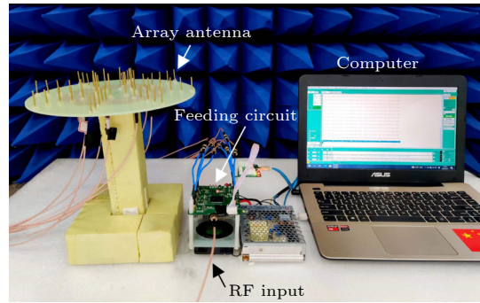
图 10 天线系统实物图
