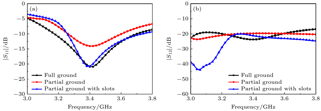
图 3 三种八木圆形阵列天线的 (a) 回波损耗和 (b) 相邻阵元隔离度
