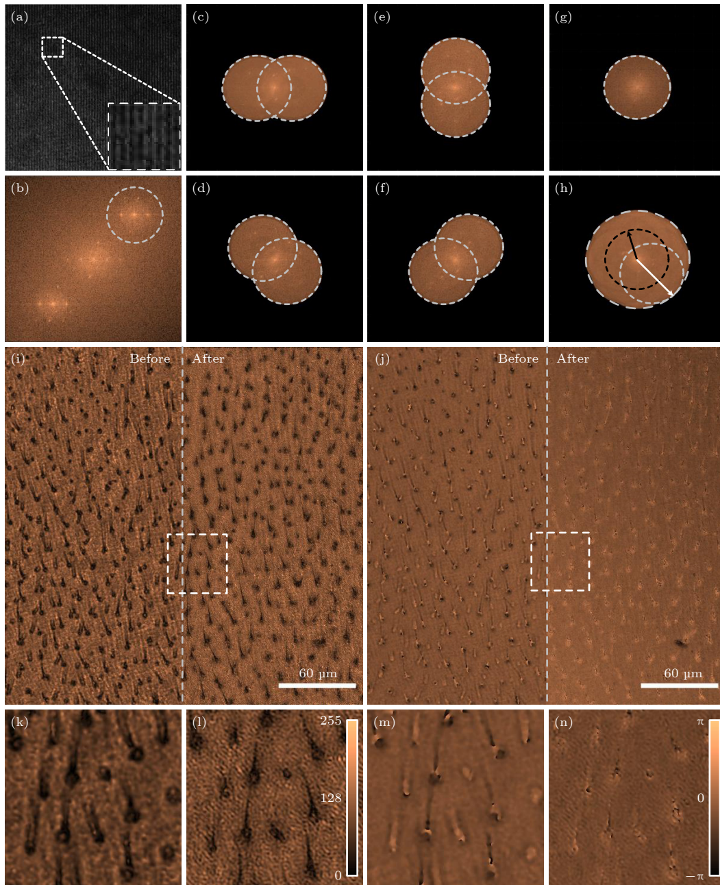
图 2 结构光照明显量相位显微的图像重构以及对苍蝇翅切片的成像结果 (a) 结构光照明显量数字全息显微的全息图; (b) 图 (a) 中全息图的频谱分布; (c)–(f) 条纹方向为 0^\circ , 45^\circ , 90^\circ 和 135^\circ 的结构光照明下得到的物光频谱分布; (g) 和 (h) 平行光照明和结构光照明下的样品频谱分布; (i) 和 (j) 苍蝇翅切片的振幅图和相位图, 其中左/右半部分别为使用平行光照明/结构光照明对应的图像; (k) 和 (l) 图 (i) 中虚框部位在平行光照明和结构光照明下恢复的振幅结果; (m) 和 (n) 图 (j) 中虚框部位在平行光照明和结构光照明下恢复的相位结果
